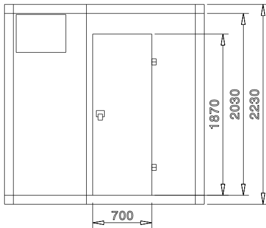
Zij aanzicht
